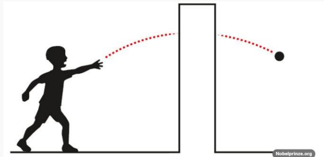
Ilustración del asombroso efecto túnel cuántico
